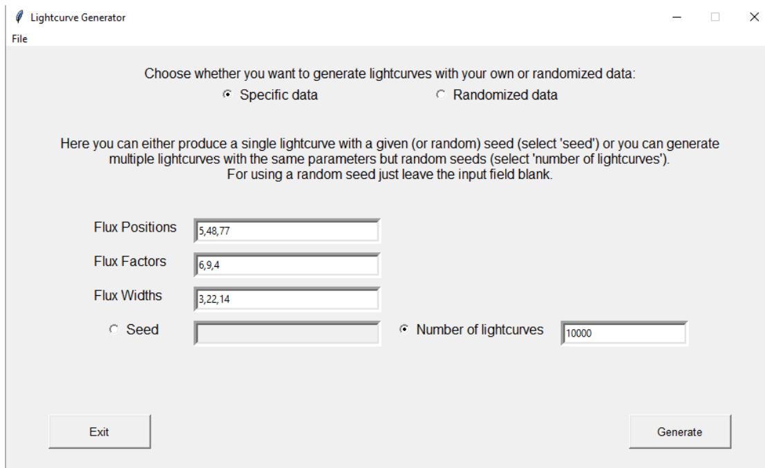
Fig. 3.1: GUI des Lightcurve-Generators. Dieses Schaubild zeigt eine Konfiguration zur Generierung von 10000 Lichtkurven. Jede einzelne von ihnen wird an den Indizes 5, 48 und 77 Strahlungsausbrüche aufweisen, wobei der Peak des Ersten 6-fach, des Zweiten 9-fach und des Dritten 4-fach größer als das Grundrauschen sein wird. Des weiteren werden diese Fluxes Halbwertsbreiten von 3, 22 und 14 Datenpunkten besitzen.
