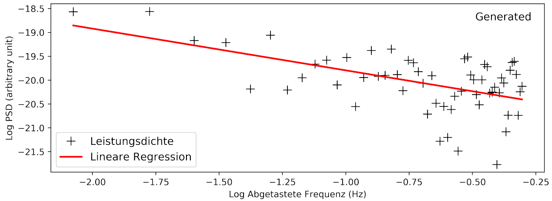
Fig. 4.9: Analoges PSD der generierten Lichtkurve aus Figur 4.4. Die Steigung beträgt hier m = -0.876 \pm 0.175 .
