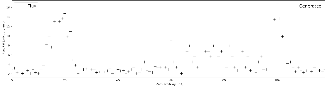
Fig. 5.6: Die aus Figur 4.4 generierte Lichtkurve, hier mit baseline = 2 .
