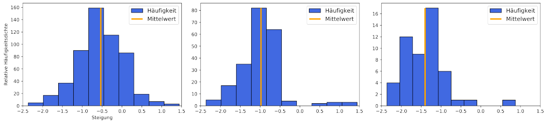
Fig. 4.7: Während im linken Histogramm alle Steigungen enthalten sind, zeigt das Mittlere nur die mit R^2 \geq 0.2 und das Rechte R^2 \geq 0.5 . Die orange Linie markiert jeweils den Mittelwert aller Slopes.
