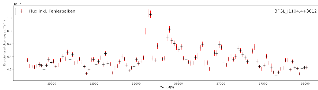
Fig. 2.3: Lichtkurve des Blazars Markarian 421
