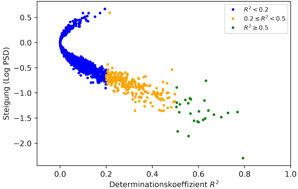
Fig. 5.2: Verwendung von 50 Zufallswerten pro Normalverteilung (im Unterschied zu Figur 4.10). Die Steigungen der Slopes sind hier eher gering und demnach im blauen Bereich konzentriert.
