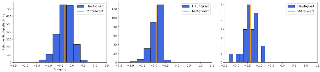
Fig. 5.3: Histogramm der generierten Lichtkurven mit 50 Zufallswerten pro Normalverteilung. Eine Filterung analog zu Figur 4.11 ergibt hier Mittelwerte von mean = -0.293 \pm 0.183 (links), mean_{0.2} = -0.898 \pm 0.168 (Mitte) und mean_{0.5} = -1.382 \pm 0.149 (rechts).
