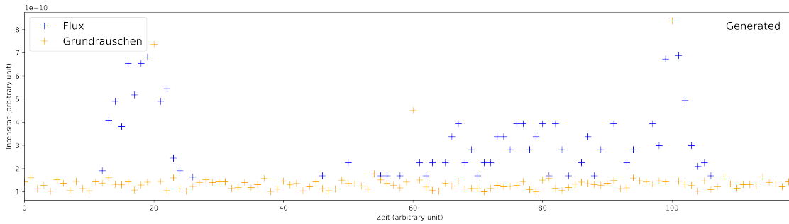
Fig. 4.4: Die orangenen Punkte in der generierten Lichtkurve stellen das ursprüngliche Grundrauschen dar. Die anschließend integrierten Fluxes sind in Blau dargestellt. Die fertige Lichtkurve enthält ausschließlich alle blauen Punkte und die orangenen, die nicht von einem blauen überlagert wurden (Figur 5.6). Der Ausbruch um die Zeit 15 bis 25 entstammt dem Histogramm aus Figur 4.3.
