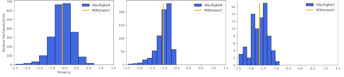
Fig. 4.11: Histogramm der generierten Lichtkurven: Analog zu Figur 4.7 sind links alle Steigungen enthalten, in der Mitte wurde nach R^2 \geq 0.2 und rechts nach R^2 \geq 0.5 gefiltert.
