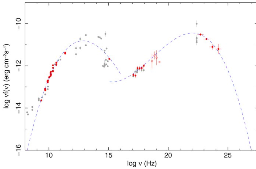
Fig. 2.2: Spektrale Energieverteilung des Blazars 4C29.45 (Abdo, Ackermann, Agudo et al., 2010).
