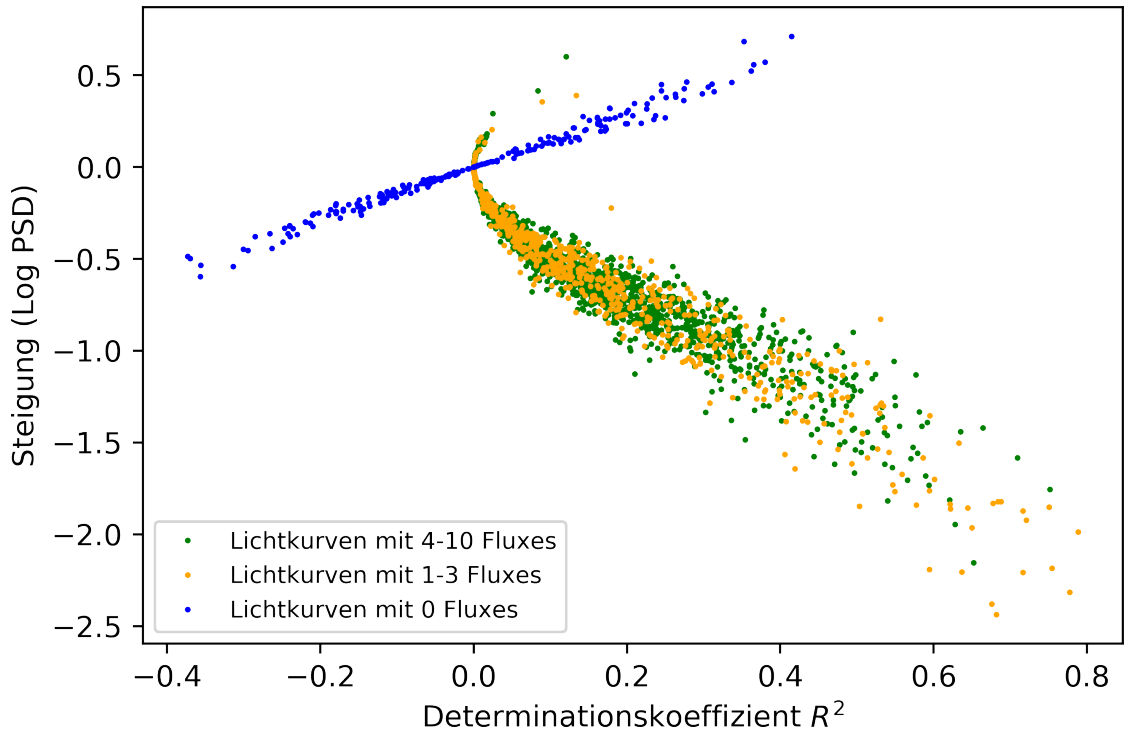
Fig. 5.7: Die blauen Punkte markieren alle Lichtkurven mit 0 Ausbrüchen, in Orange die mit 1-3 und in Grün die mit 4-10. Es ist zu beachten, dass die Grafik 1453 grüne und 614 orangene Datenpunkte zeigt.
