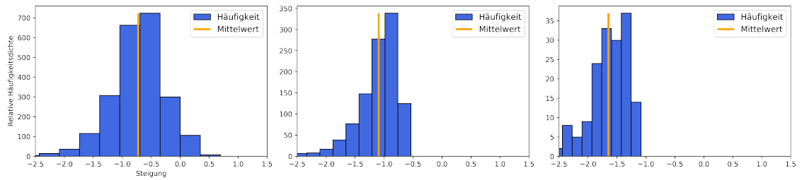
Fig. 5.5: Histogramm der generierten Lichtkurven mit 500 Zufallswerten pro Normalverteilung. Nach der Filterung ergeben sich die Mittelwerte zu mean = -0.726 \pm 0.196 (links), mean_{0.2} = -1.095 \pm 0.189 (Mitte) und mean_{0.5} = -1.648 \pm 0.178 (rechts).
