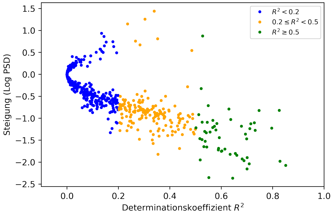
Fig. 4.8: Die nur schwach korrelierten Steigungen weisen größtenteils Werte zwischen -1 und +1 auf. Je stärker die Korrelation wird, desto weiter fällt die mittlere Steigung ab.
