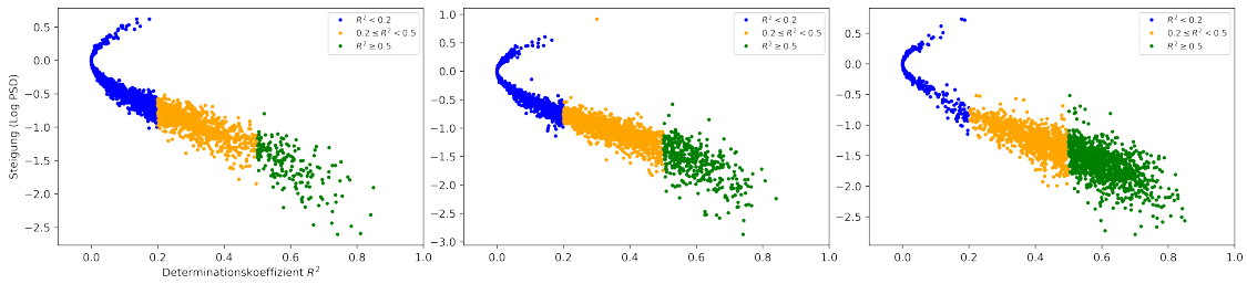
Fig. 5.10: Alle drei Grafiken zeigen die Verteilung der Steigungen im PSD von 2278 zufällig generierten Lichtkurven. Links wurde die maximale Breite auf 75 Datenpunkte begrenzt, in der Mitte auf 50 und rechts auf 25.
