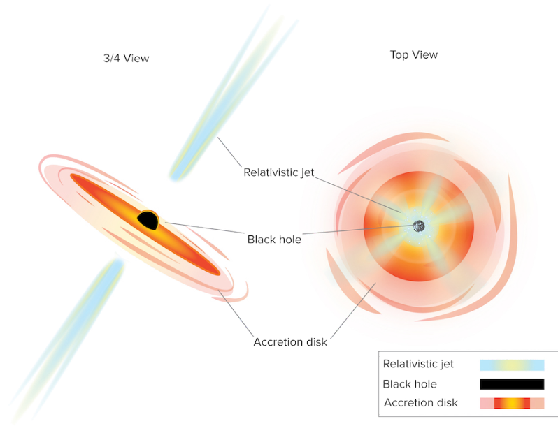
Fig. 2.1: Aufbau eines Blazars (Dagnello, o. J.)
