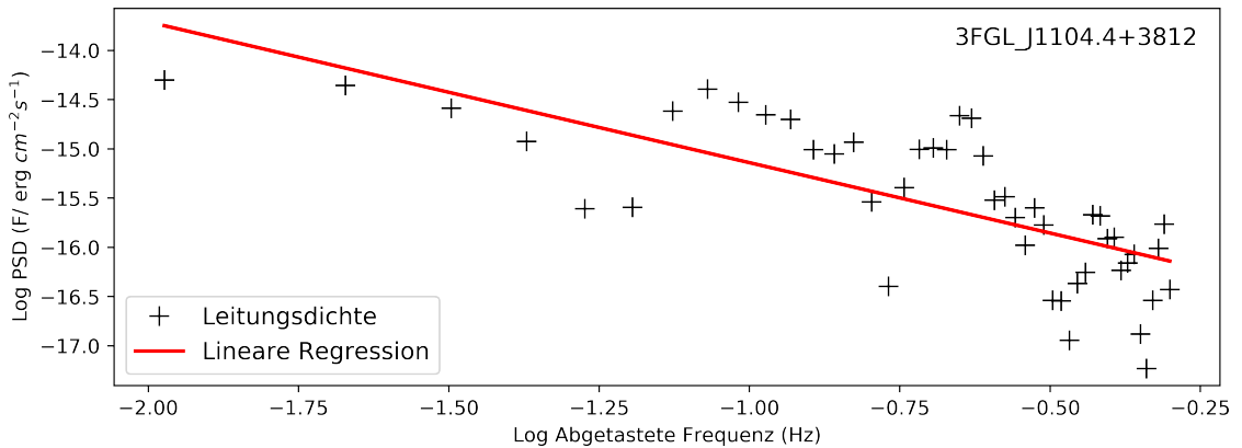
Fig. 5.1: Leistungsdichtespektrum des Blazars Markarjan 421. Im Gegensatz zu Figur 4.5 werden hier nur die 94 signifikantesten Datenpunkte einbezogen. Die Steigung beträgt hier m = -1.429 \pm 0.205 .
