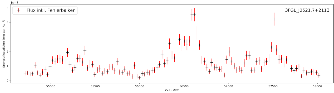
Fig. 4.1: Lichtkurve der Quelle TXS 0518+211: Um die Zeit 56000 baut sich der Peak allmählich auf und fällt extrem schnell ab, während bei 57500 sowohl Anstieg als auch Abfall rasant sind.
