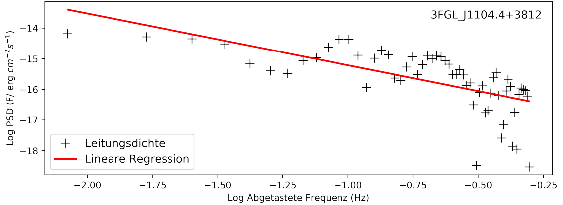
Fig. 4.5: Leistungsdichtespektrum des Blazars Markarjan 421 (Lichtkurve siehe Figur 2.3). Die Steigung der ausgleichenden Geraden (rot) beträgt m = -1.688 \pm 0.253 .
