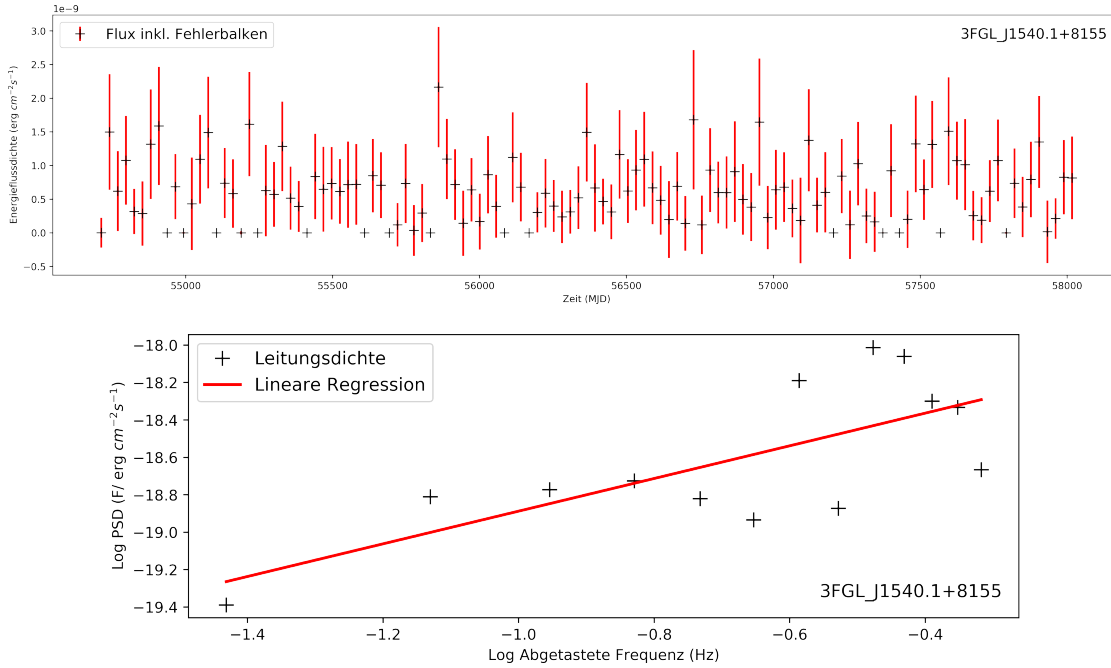
Fig. 4.6: Lichtkurve (oben) und Leistungsdichtespektrum (unten) des BL Lac-Blazars 1ES 1544+820 mit mittlerer Steigung m = 0.873 \pm 0.249 .
