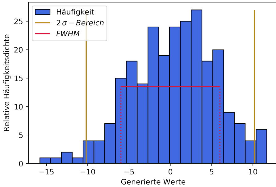
Fig. 4.3: Histogramm mit \mu = 0 und Flux-Width = FWHM = 12. Nach Formel (4.3) erhält man bins = 20.4 , was auf bins = 21 aufgerundet wird. Die beiden beige Linien markieren den 2\sigma -Bereich. Die horizontale, rote Linie repräsentiert die Halbwertsbreite auf halber Höhe des Maximums.
