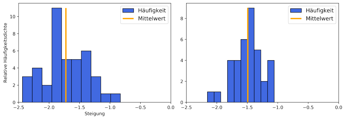
Fig. 5.8: In diesen Histogrammen ist klar zu erkennen, dass nach einer Filterung von R^2 \geq 0.5 die Steigungen bei 1-3 Fluxes (links, mean_{1-3} = -1.725 \pm 0.180 ) deutlich steiler sind als bei 4-10 Fluxes (rechts, mean_{4-10} = -1.492 \pm 0.171 ).
