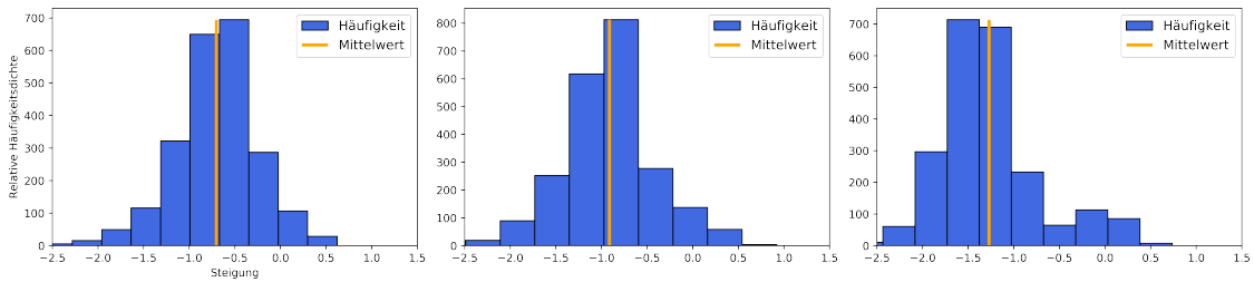
Fig. 5.11: Bei \text{FWHM} \leq 75 erzielt man \text{mean}_{\text{gen},75} = -0.703 \pm 0.193 (links), bei \text{FWHM} \leq 50 beträgt er \text{mean}_{\text{gen},50} = -0.913 \pm 0.192 und \text{FWHM} \leq 25 zeigt \text{mean}_{\text{gen},25} = -1.272 \pm 0.189 .
