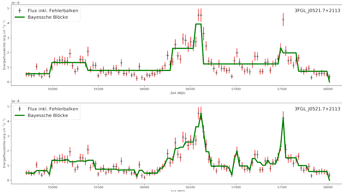
Fig. 4.2: Lichtkurven der Quelle TXS 0518+211: Anwendung der bayesschen Blöcke (nach Scargle) mit \sigma = 5.0 \cdot 10^{-9} \text{ erg cm}^{-2} \text{ s}^{-1} (oben) und \sigma = 1.0 \cdot 10^{-9} \text{ erg cm}^{-2} \text{ s}^{-1} (unten).
