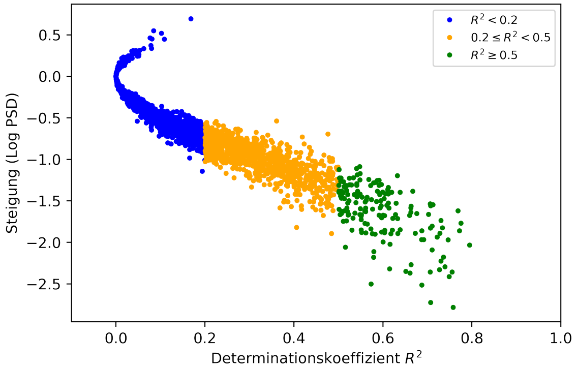
Fig. 5.4: Verwendung von 500 Zufallswerten pro Normalverteilung. Im Vergleich zu Figur 4.10 sind die Steigungen der Slopes hier eher steiler orientiert und demnach im orangen/grünen Bereich.
