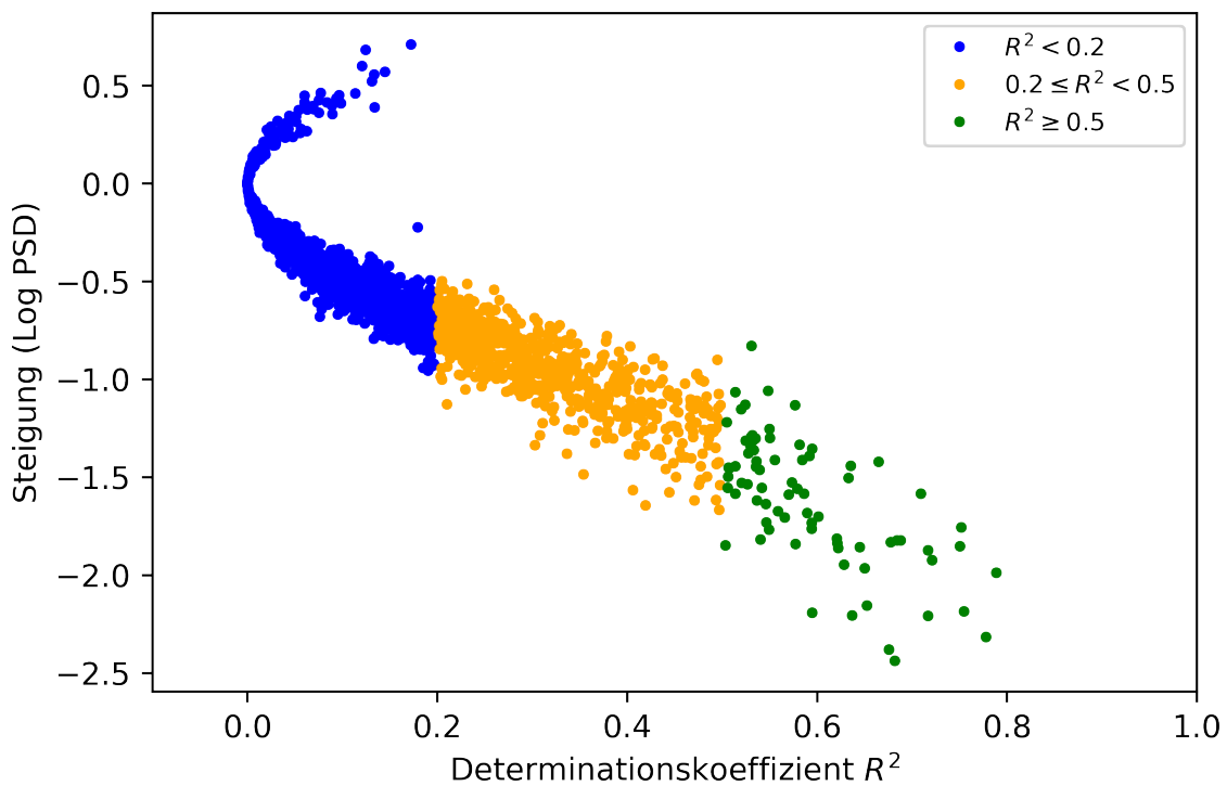
Fig. 4.10: Steigung zu Determinationskoeffizient für die zufällig generierten Quellen: Die Verteilung ist nahe zu identisch zu der in Figur 4.8 (reale Quellen), jedoch sind die Steigungen für jedes R^2 geringer gestreut.
