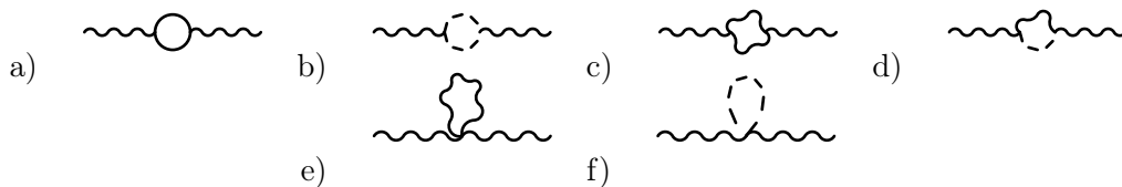
Abbildung 2.4: 1-Loop Graphen der Vektor-Wellenfunktion ohne Tadpoles
