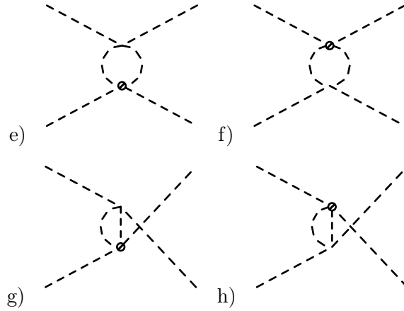
Abbildung 3.13: 1-Loop-Korrekturen durch quartische Wechselwirkungen.
