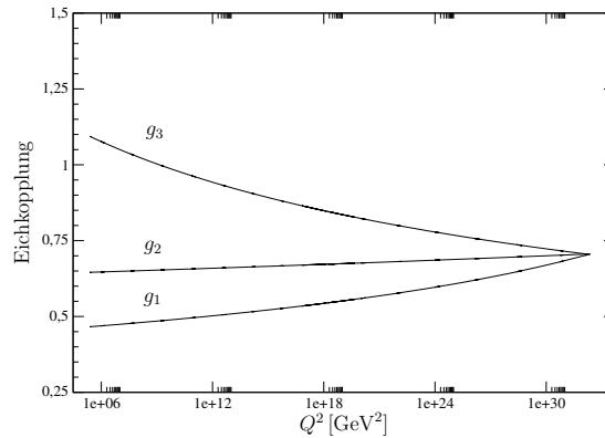
Abbildung 1.2: Vereinigung der Eichkopplungen bei SUSY an der Planck-Skala
