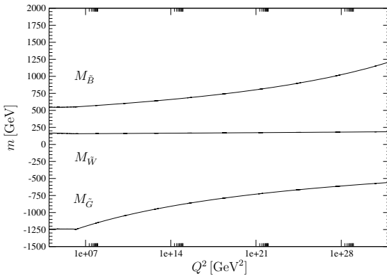
Abbildung 4.9: Gauginomassen für den SPS-Punkt 9 (AMSB)
