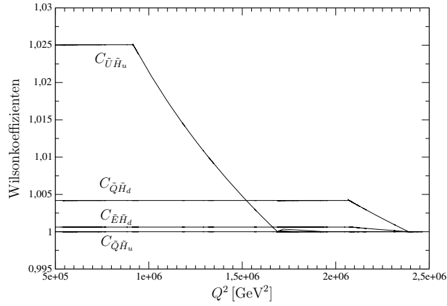
Abbildung 4.19: Entwicklung einiger Wilsonkoeffizienten beim SPS 2
