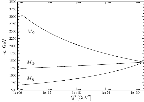
Abbildung 4.5: Gauginomassen für den SPS-Punkt 2 (mSugra)
