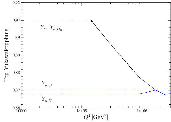
Abbildung 4.18: Unterschied zwischen den Top Yukawakopplungen beim SPS 2
