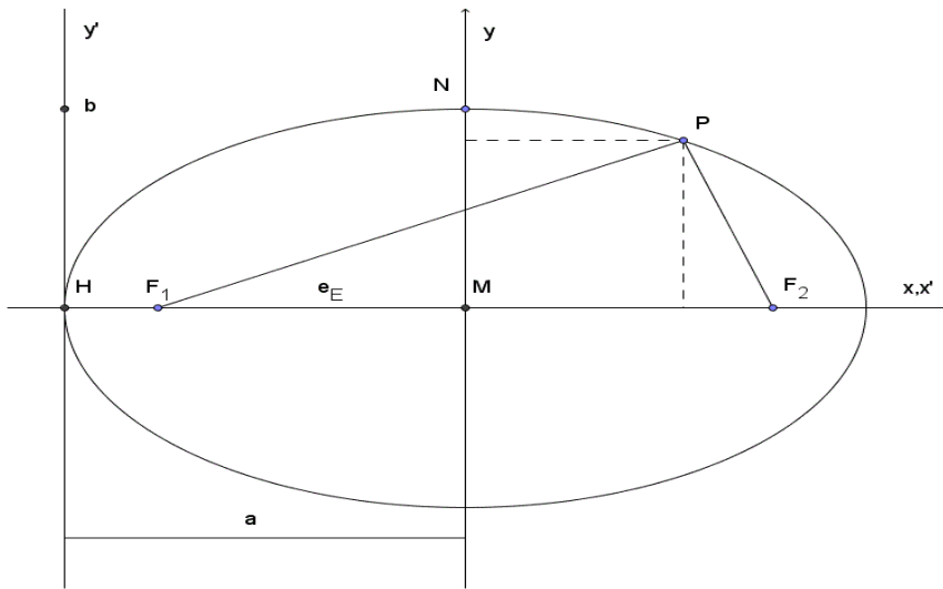
Abb. 1: Zur Mittelpunktsgleichung und Scheitelgleichung der Ellipse
