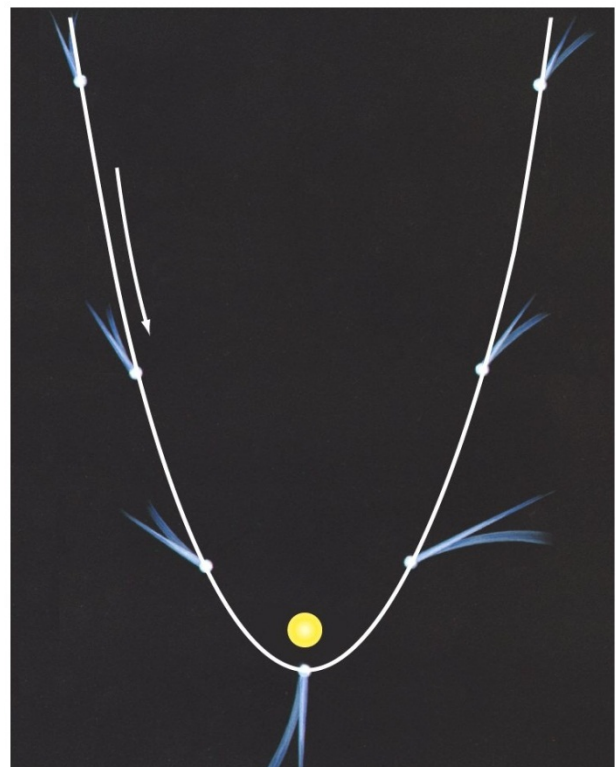
Abb. 3: Komet beim Umlauf um die Sonne
